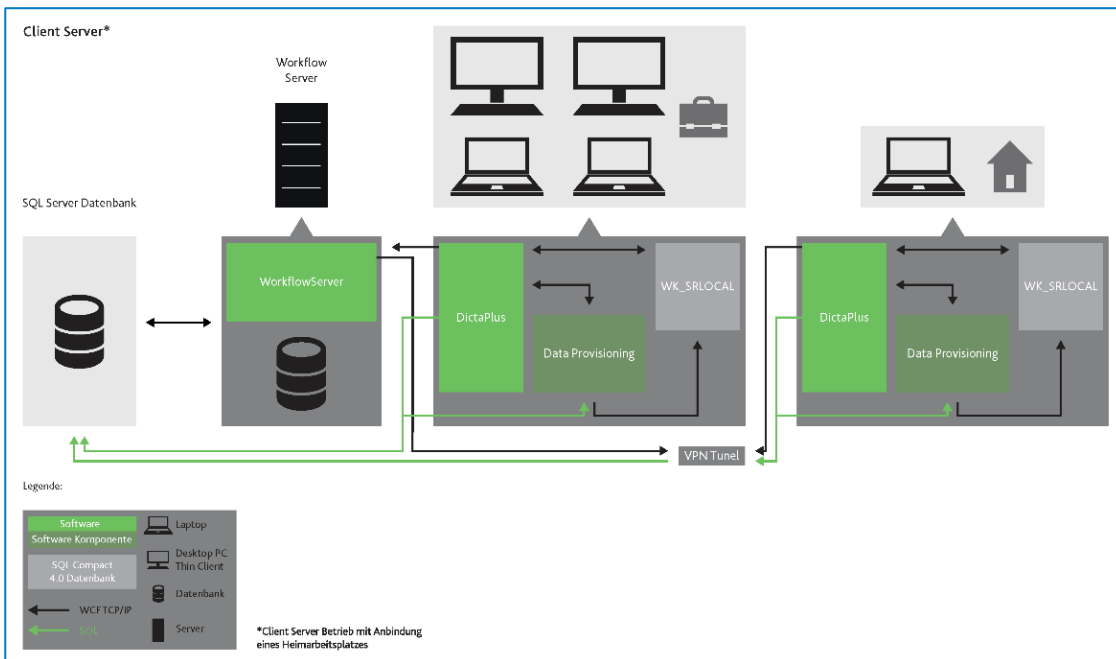
Abbildung 4: Client Server mit Remote Arbeitsplatz
