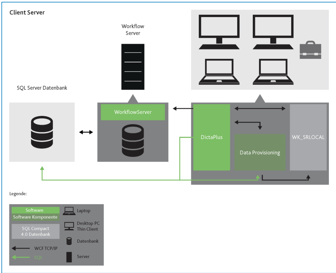
Abbildung 2: Infrastruktur Client Server
