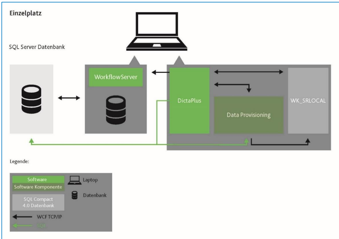
Abbildung 1: Infrastruktur Einzelplatz
