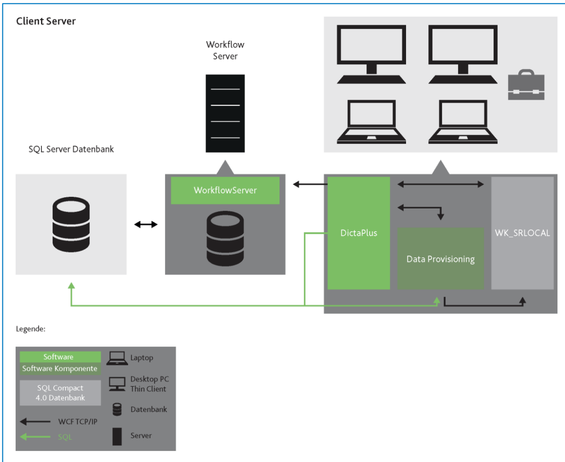
Abbildung 3: Client Server im Netzwerk
